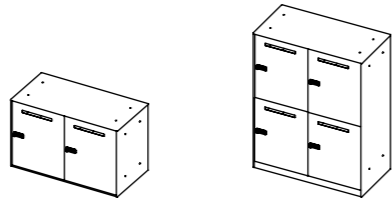
Upward 上置 W900 D450 H556.5 Base 下置 W900 D450 H1136
