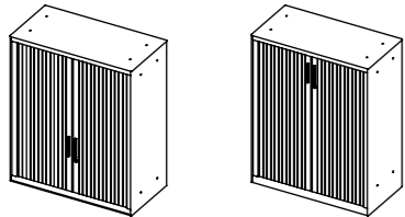
Upward 上置 W900 D450 H724/1076 Base 下置 W900 D450 H784/1136
