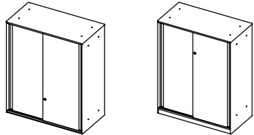
Upward 上置 W900 D450 H724/1076 Base 下置 W900 D450 H784/1136
